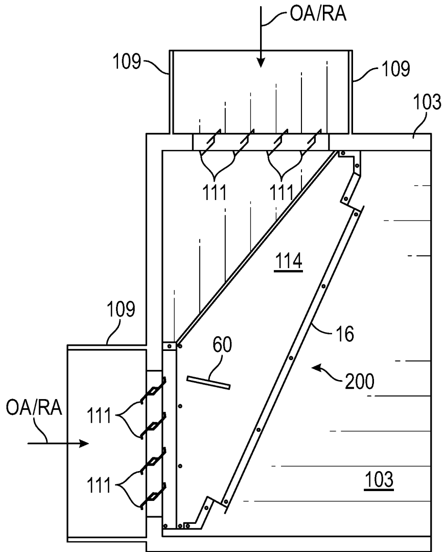
FIG. 22
