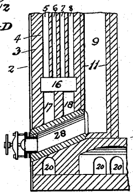
Section VIII-VIII Fig. 8
