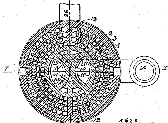
Section C-D Fig. 5
