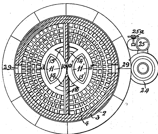
Section A-B Fig. 4
