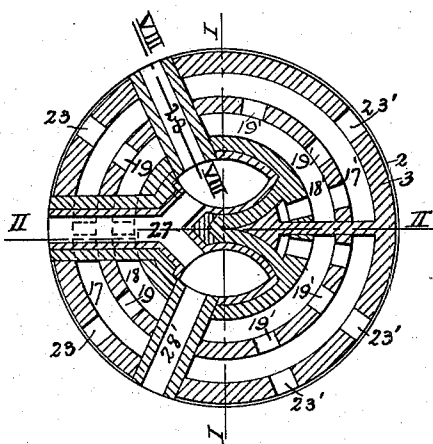
Section E-F Fig. 6
