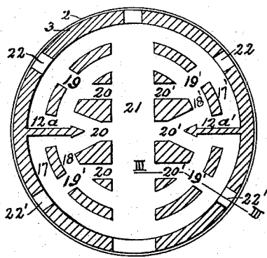
Section G-H Fig. 7
