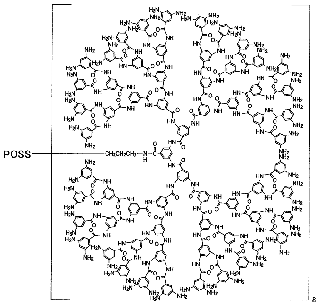
G6 Dendrimer
