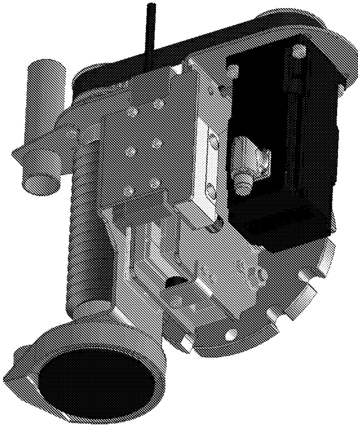
Fig. 5 Den Schleifkopf aus Fig. 2 in Ansicht von schräg unten;
