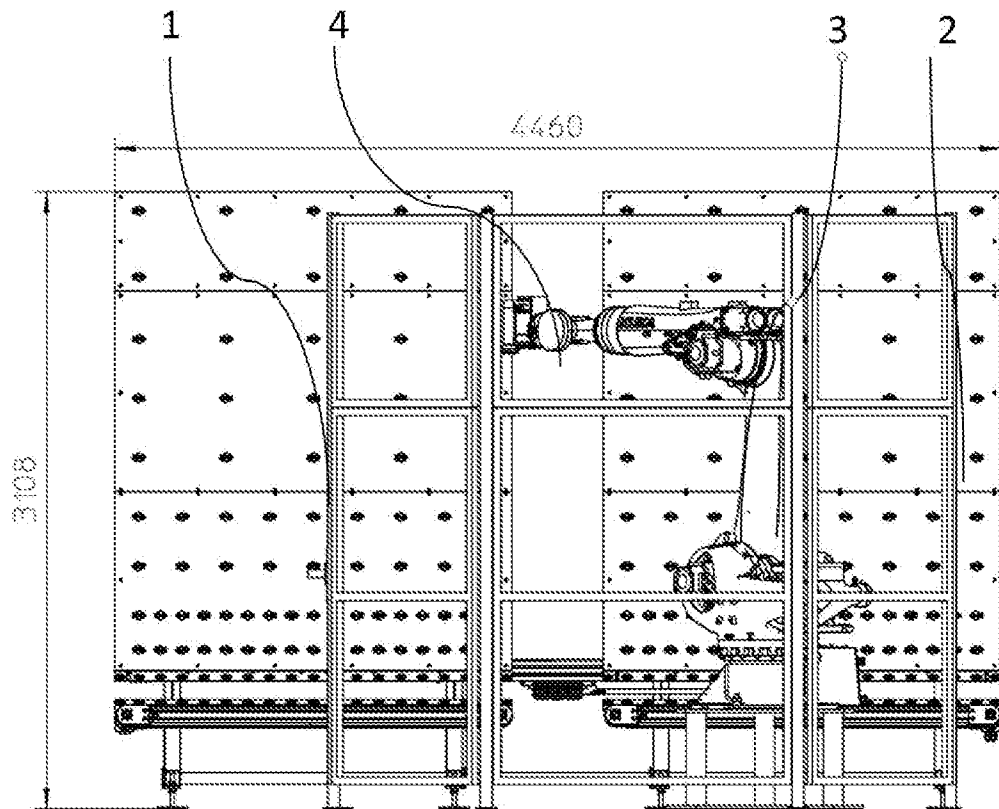
Fig. 1 Eine erfindungsgemäße Anlage mit Mehrachsenroboter in Ansicht;
