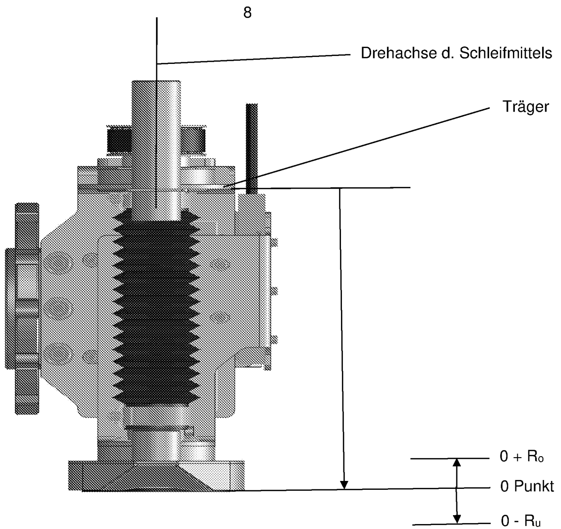
Fig. 3 Den Schleifkopf aus Fig. 2 in Vorderansicht;
