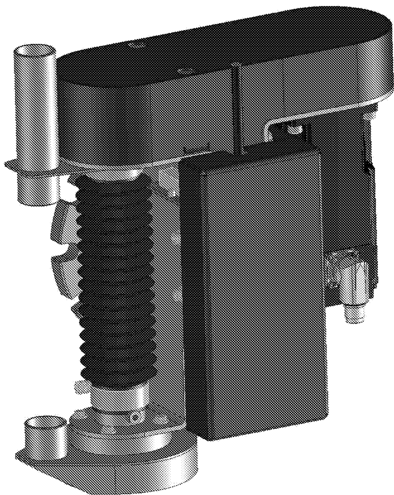
Fig. 6 Den Schleifkopf aus Fig. 2 in Schrägansicht mit Kopfabdeckungen;
