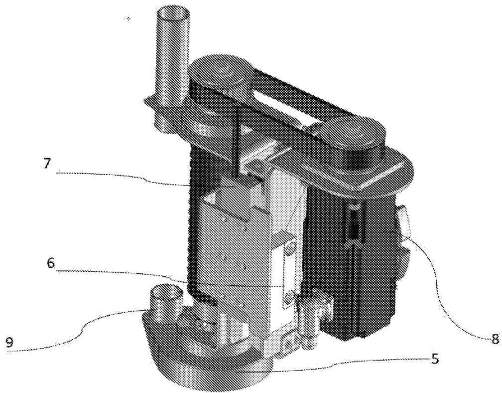
Fig. 2 Ein erfindungsgemäßer Schleifkopf in Schrägansicht;
