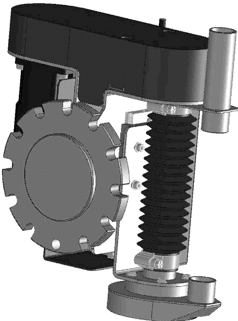
Fig. 7 Den Schleifkopf aus Fig. 6 in einer weiteren Schrägansicht;
