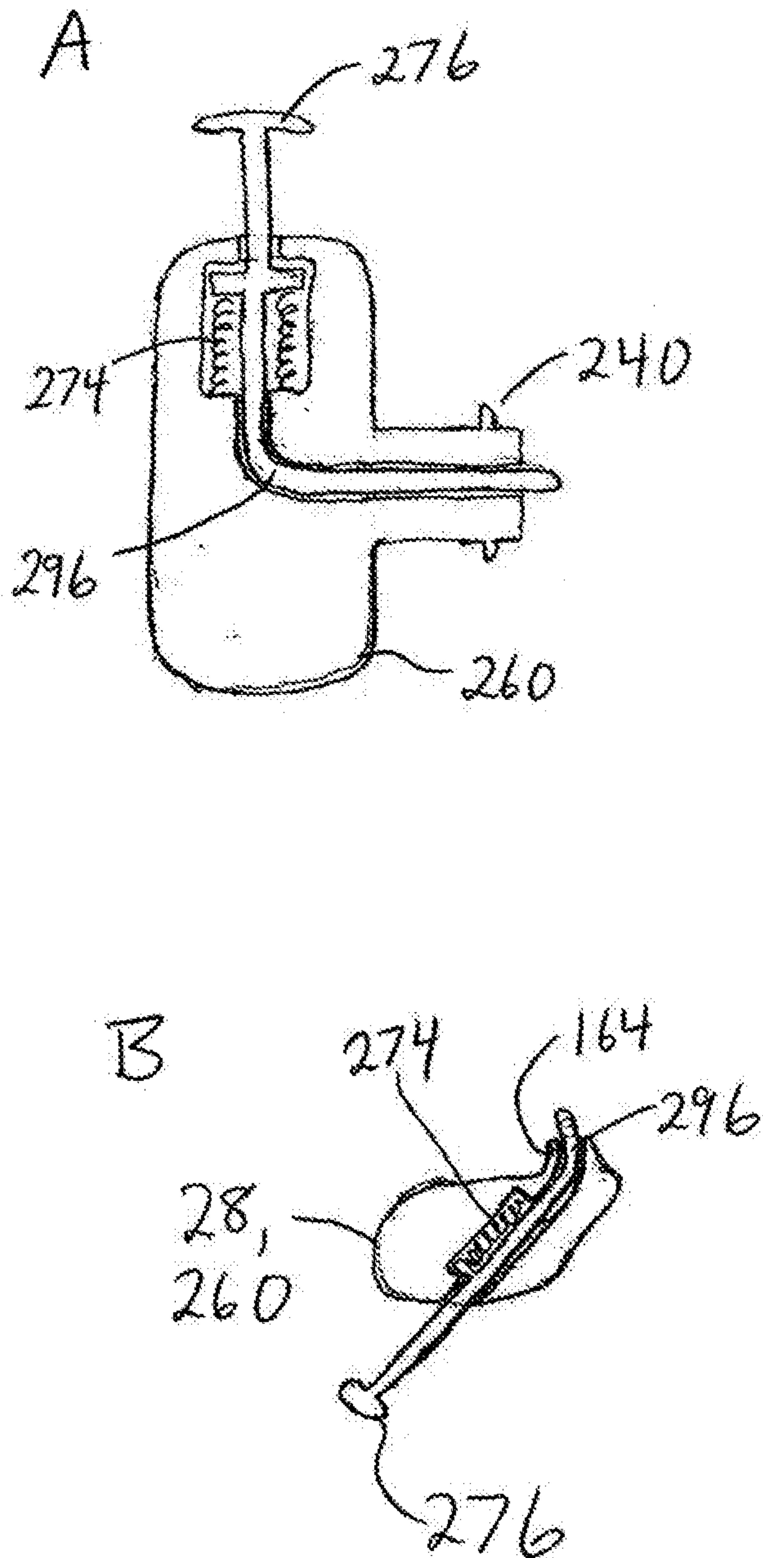
FIG. 108. Angled Push Rod
