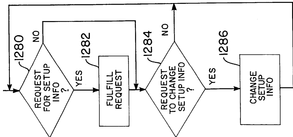
FIG. 50 SETUP MGR.
