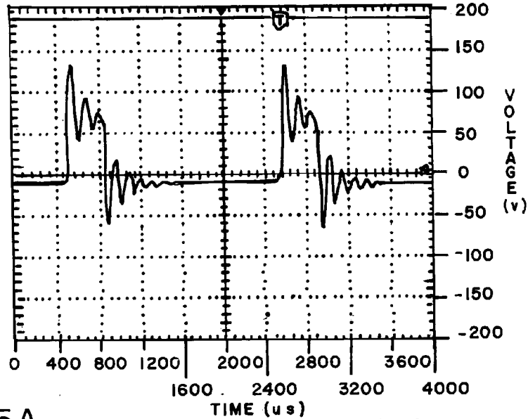
FIG.5A I-M-Ohm IMPENDANCE
