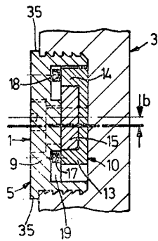
Fig.14 (VI-VI)
