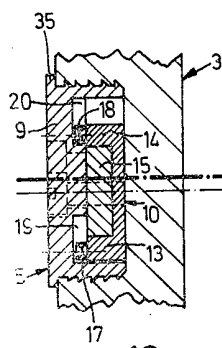
Fig. 10 (III-III)
