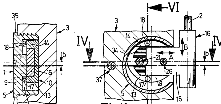
Fig.13 (V-V)
