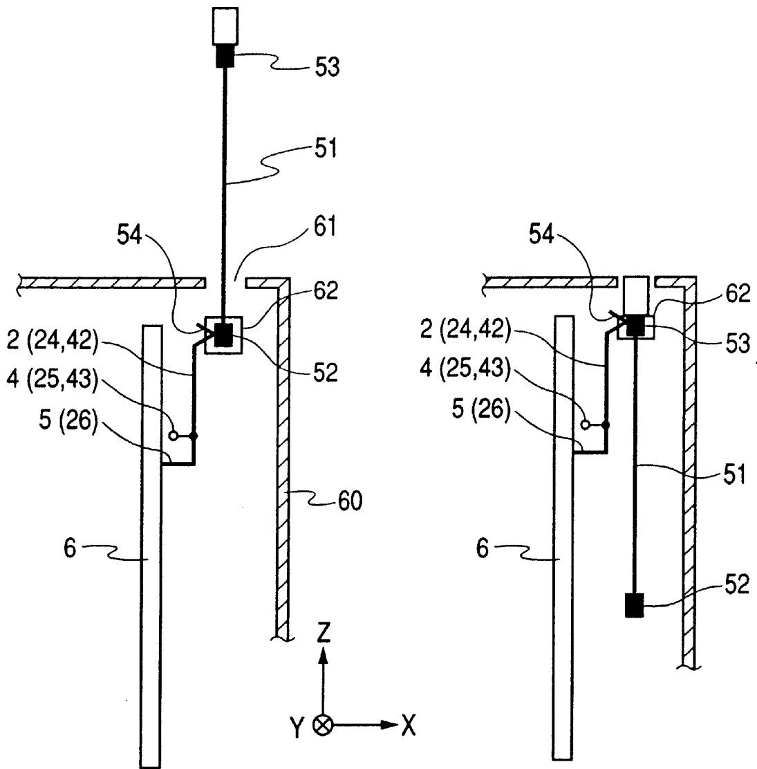
FIG. 16A
