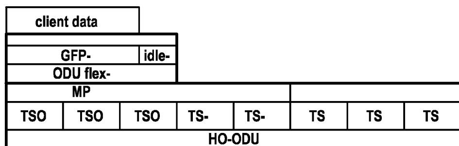
Fig. 8d
