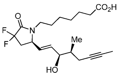
Example 1H
