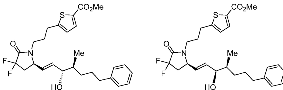
Example 28A
