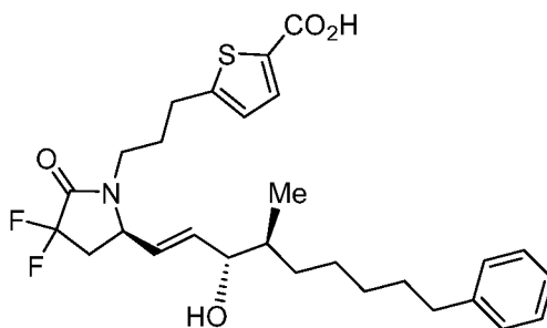
Example 39C
