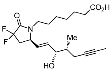
Example 1G
