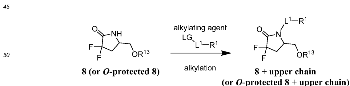
Scheme 2A
