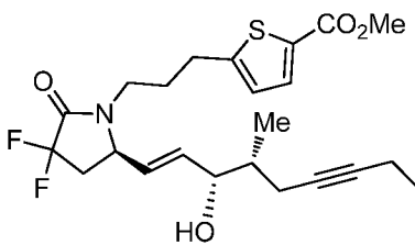
Example 24B
