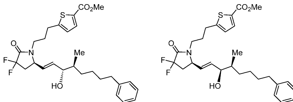
Example 38A
