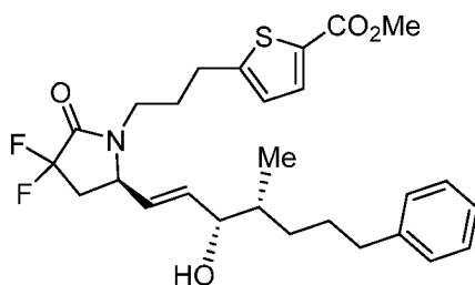
Example 28E
