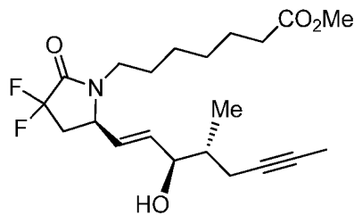
Example 1E
