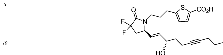
Example 32C
