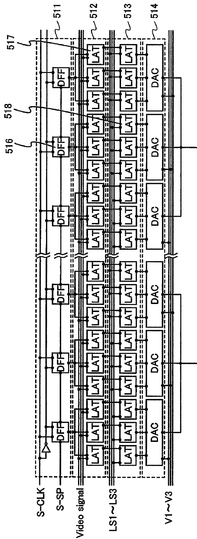
FIG. 12
