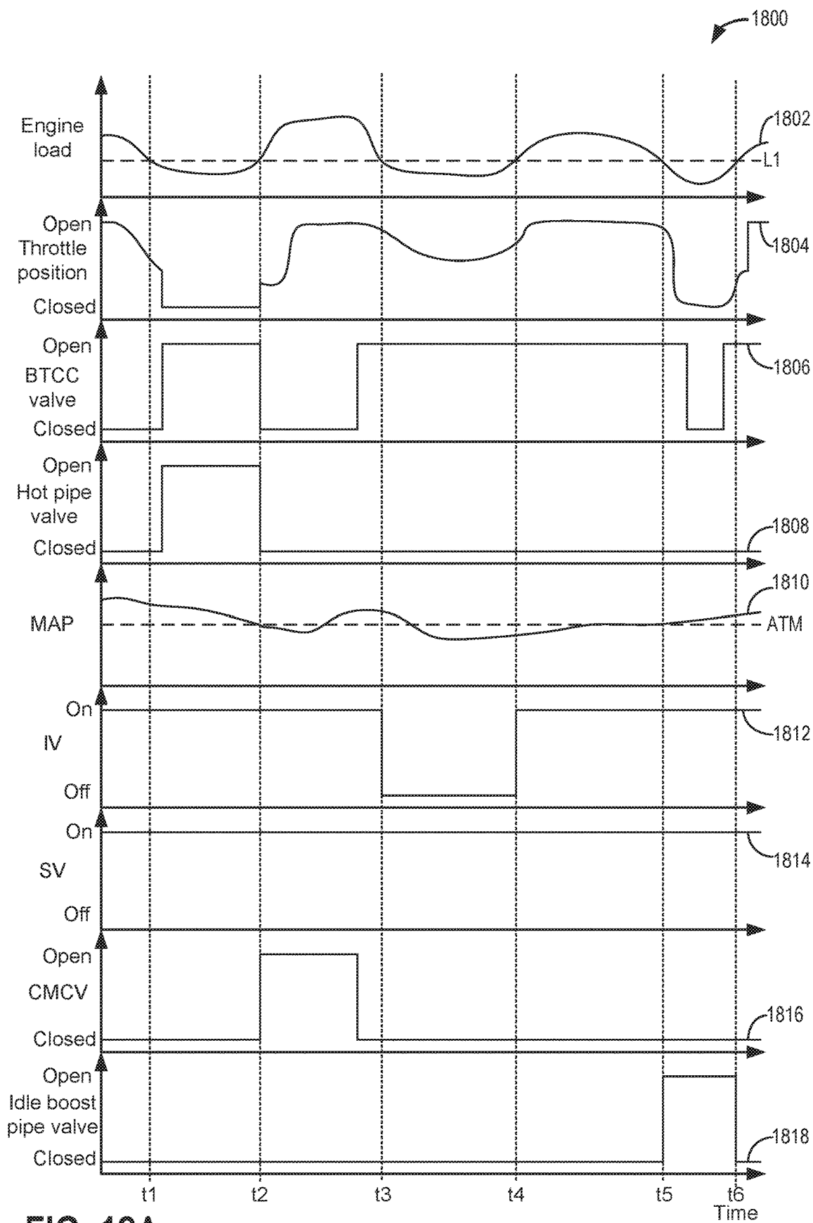
FIG. 18A
