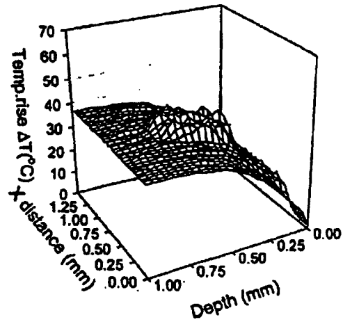
FIG. 7B6 1340 nm
