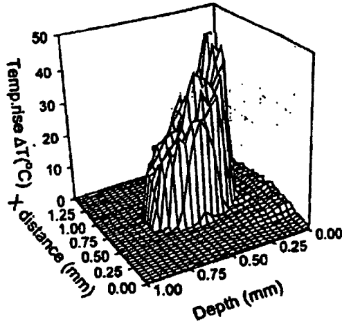
FIG. 7A5 1064 nm
