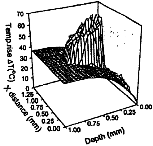
FIG. 7B5 1064 nm
