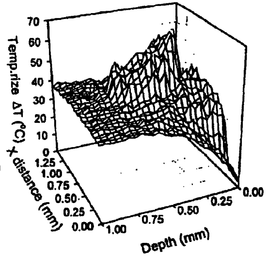
FIG. 7B7 1540 nm
