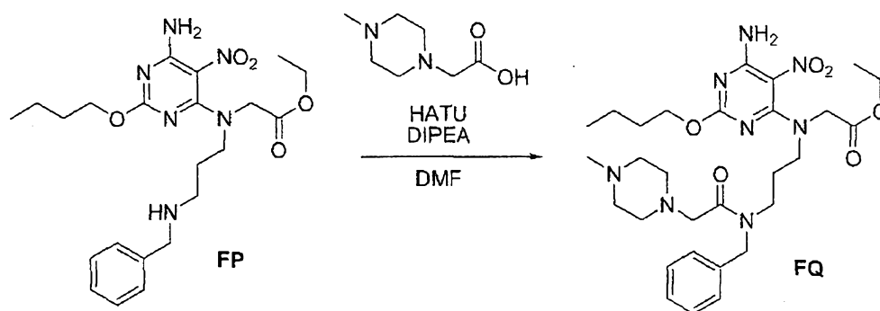
Scheme 107:
