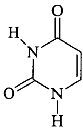
Uracil
