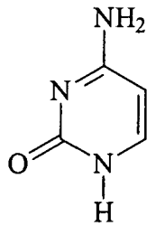
Cytosine
