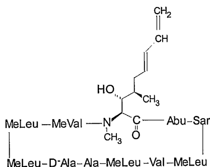
E-isomer
