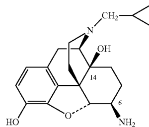
β-Naltrexamine
