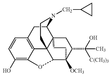
Buprenorphine
