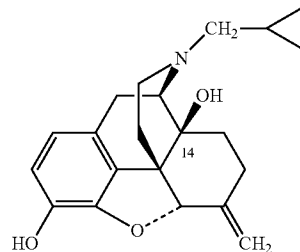
Nalmefene
