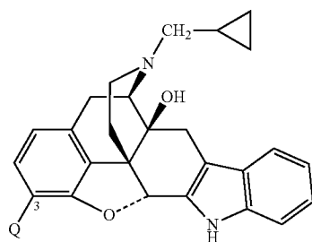
Naltrindole core
