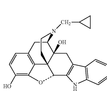
Naltrindole
