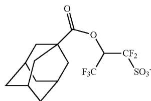
PAG1
