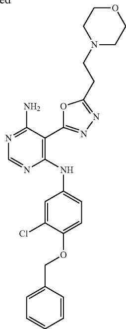
Cpd 193
