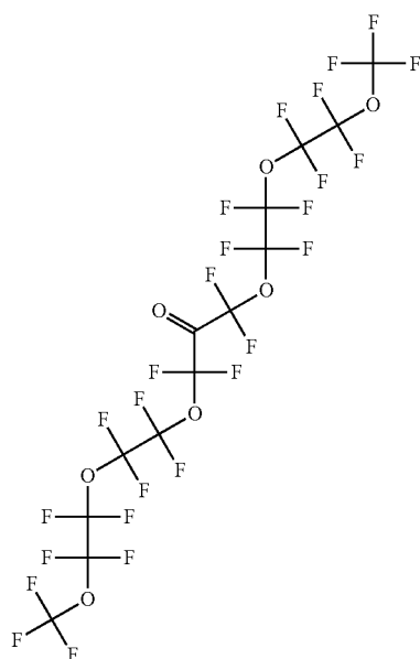
Perfluoro-3,6,9-trioxadecanoic anhydride
