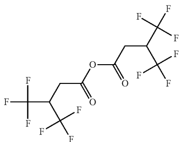
4,4,4-Trifluoro-3-(trifluoromethyl)butyric anhydride
