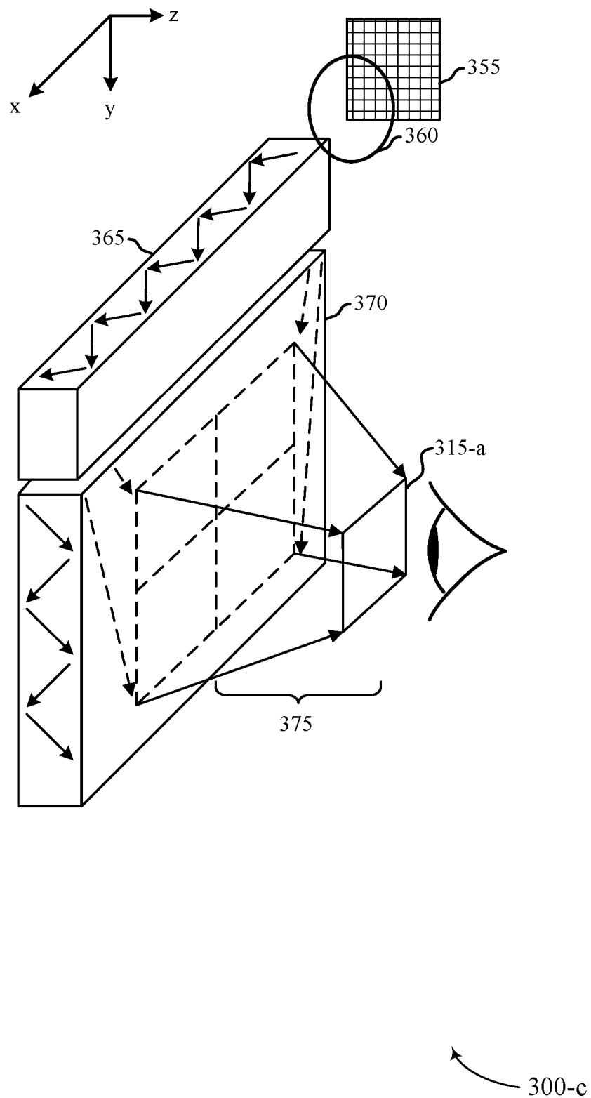
FIG. 3C
