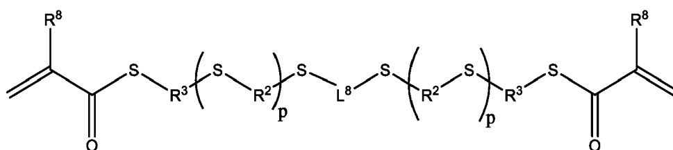
(IIg)
