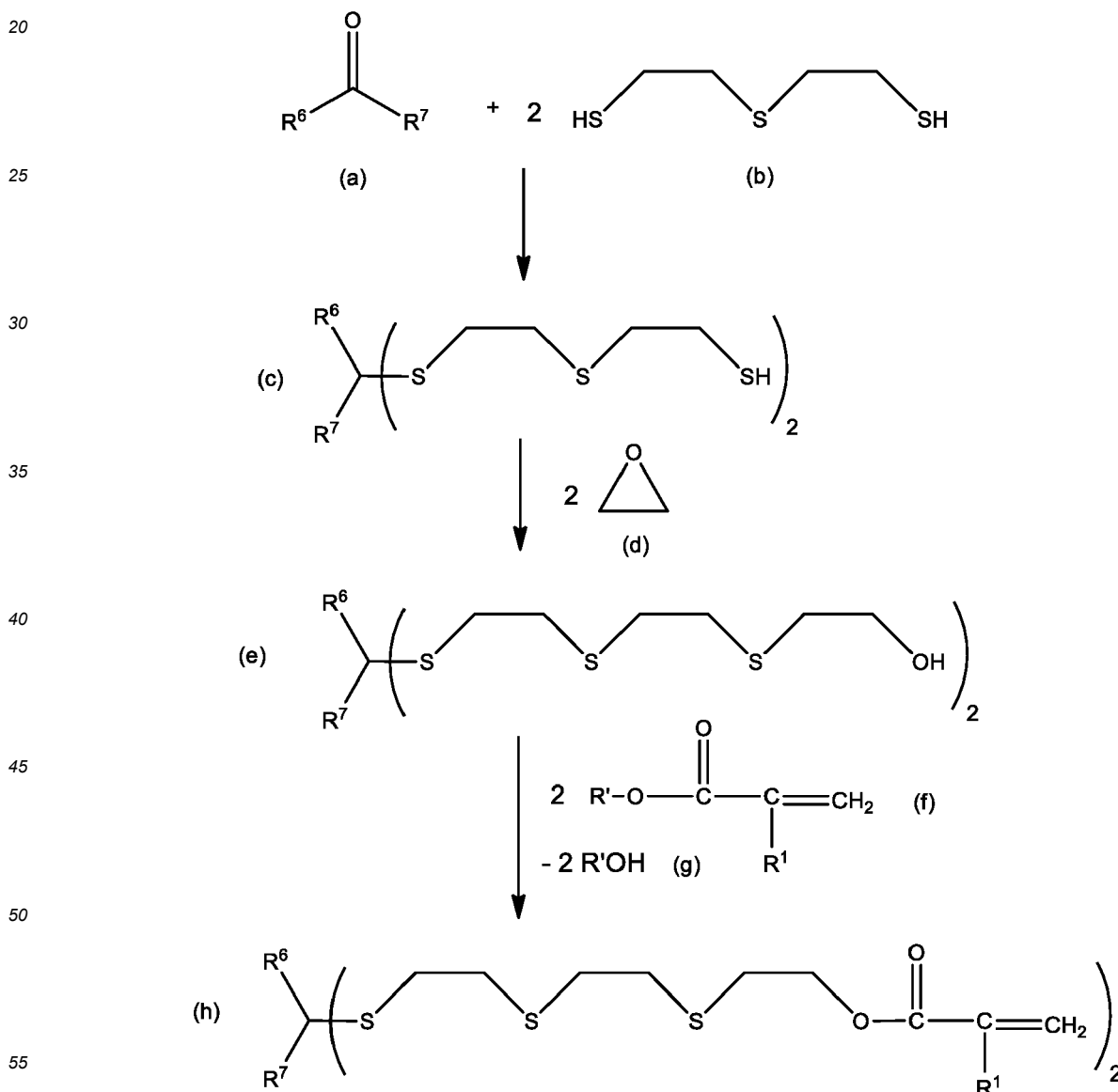
Scheme-(A)
