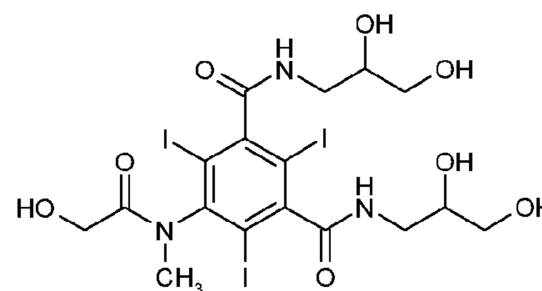
Iomeprol
