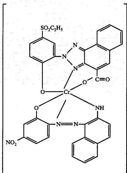
Rosinamin D-ammonium ion
