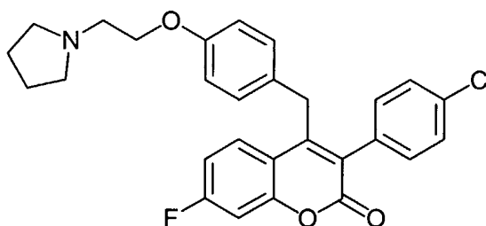
3-(4-Chloro-phenyl)-7-fluoro-4-[4-(2-pyrrolidin-1-yl-ethoxy)-benzyl]-chromen-2-one
