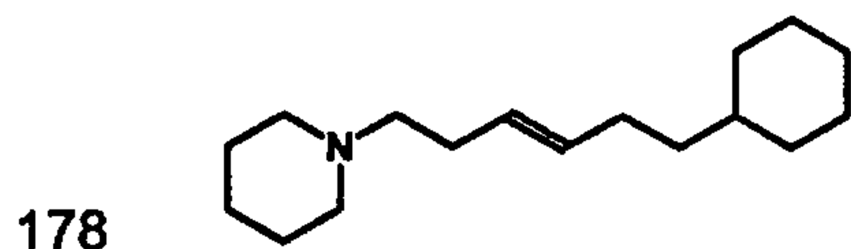
trans -1-(6-Cyclohexyl-3-hexen-1-yl)piperidine
