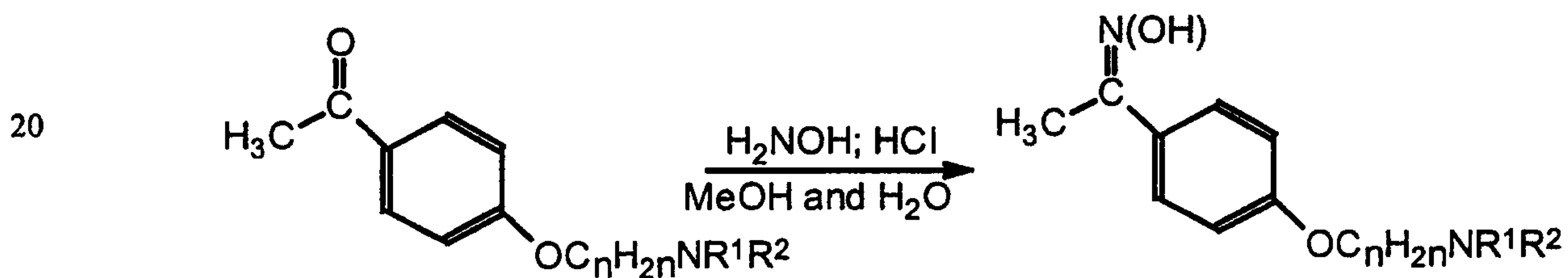
SCHEME 5 (method J):
