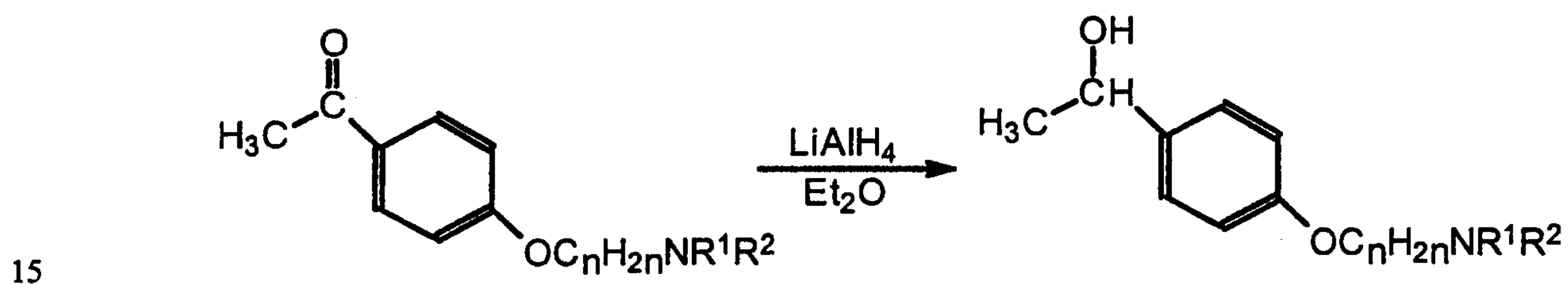
SCHEME 4 (method G):
