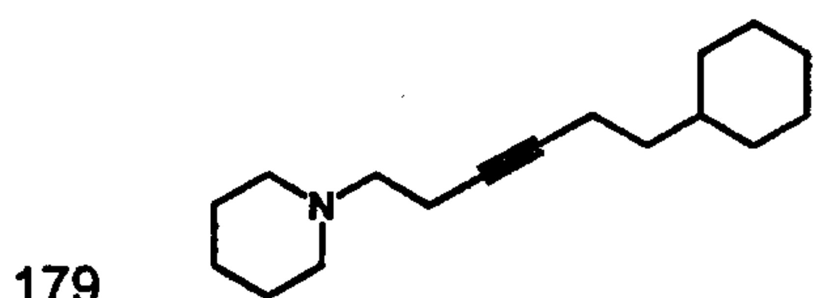
1-(6-Cyclohexyl-3-hexin-1-yl)piperidine
