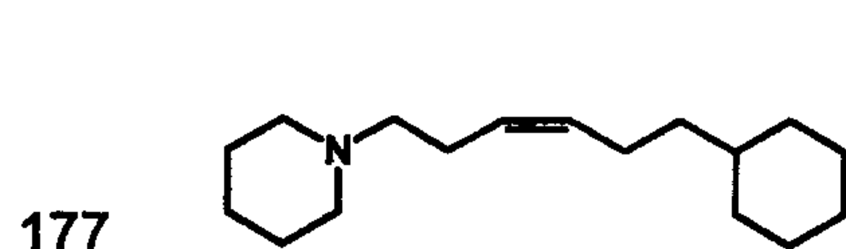
cis -1-(6-Cyclohexyl-3-hexen-1-yl)piperidine
