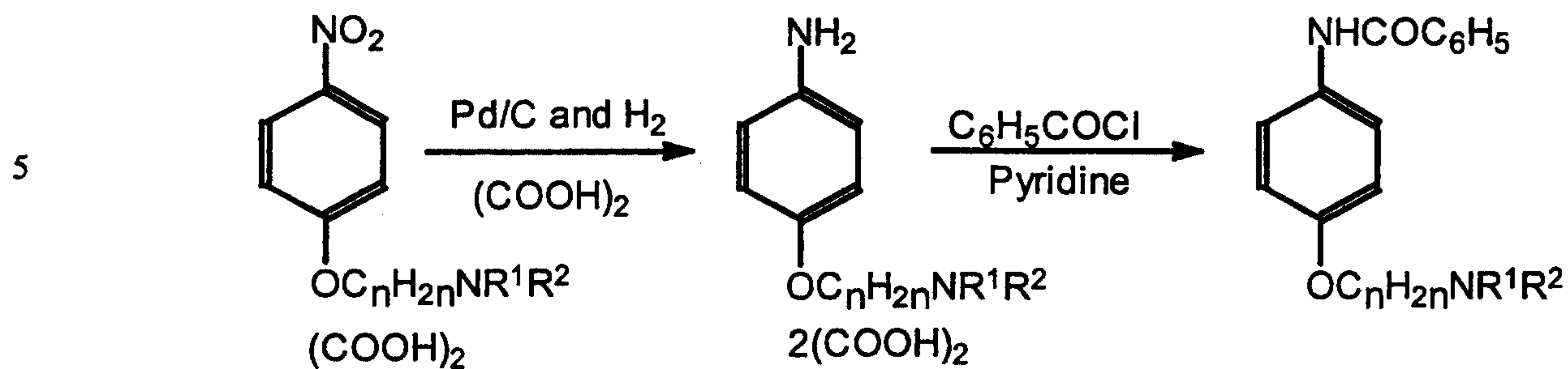
SCHEME 3 (method E):
