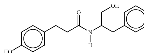
C_{18}H_{21}NO_3 Mol. Wt.: 299.36
