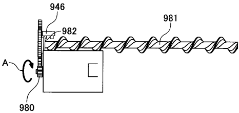
(A) 平面図
