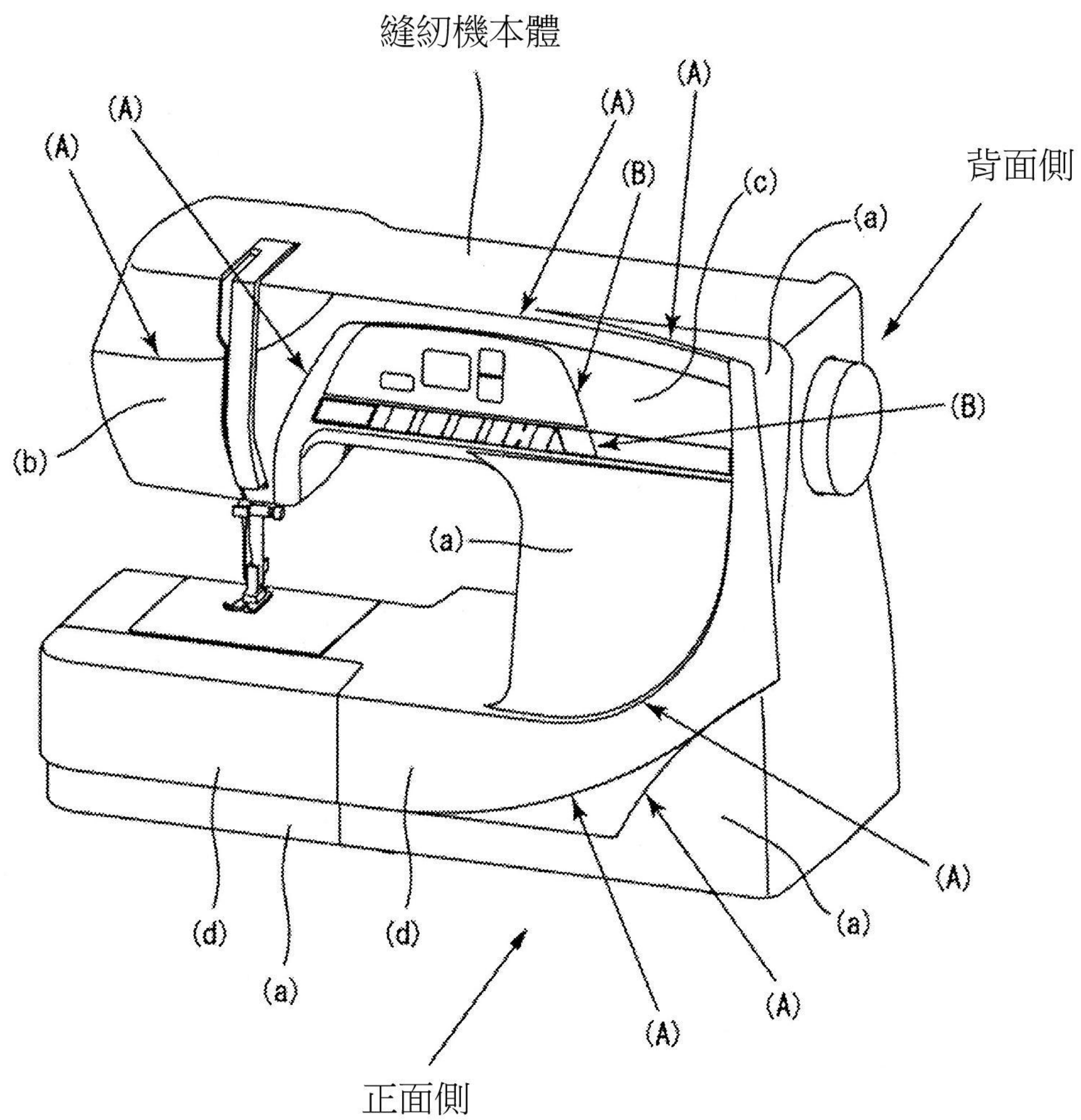
【設計說明參考圖】
