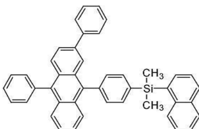
[화합물 53]
