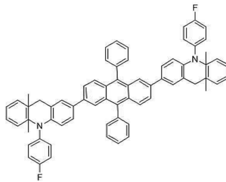
[화합물 136]
