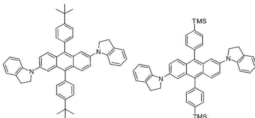
[화합물 65]
