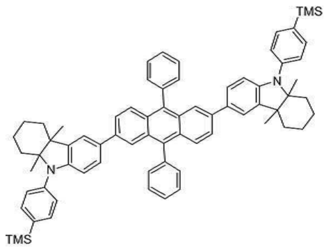
[화합물 125]
