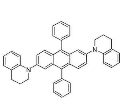
[화합물 79]
