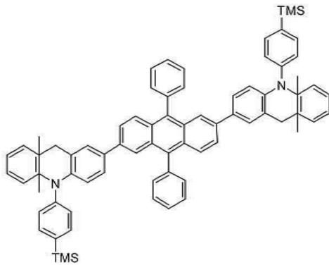
[화합물 135]
