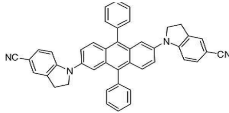
[화합물 78]
