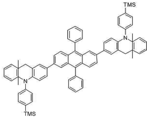
[화합물 135]
