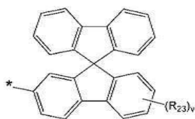
화학식 4D
