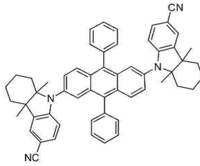
[화합물 104]
