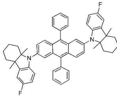
[화합물 102]
