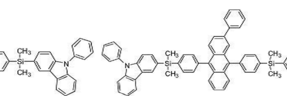
[화합물 52]
