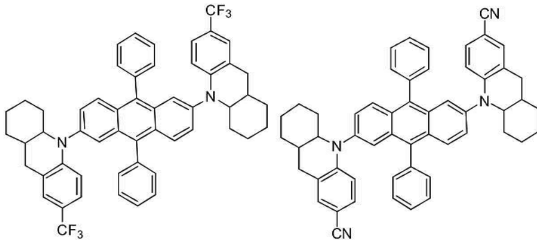
[화합물 117]
