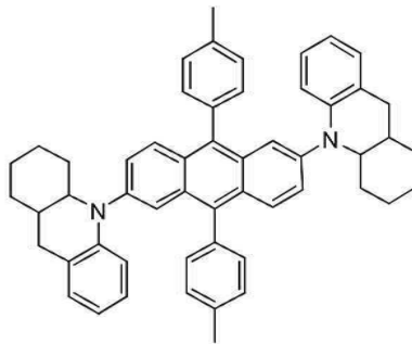
[화합물 110]
