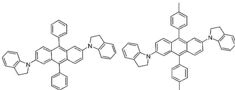
[화합물 63]
