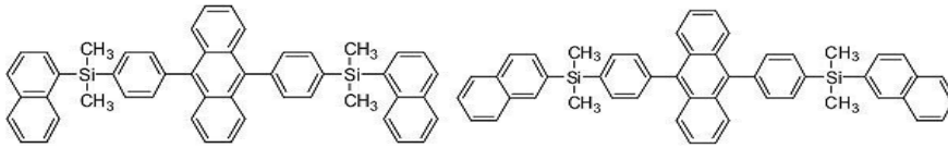
[화합물 5]
