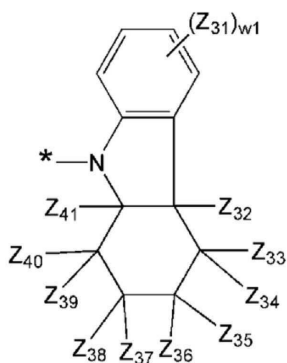
<화학식 7E>
