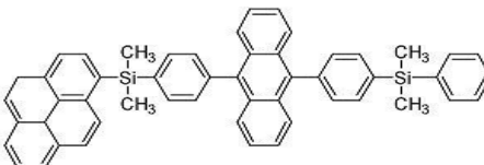
[화합물 8]
