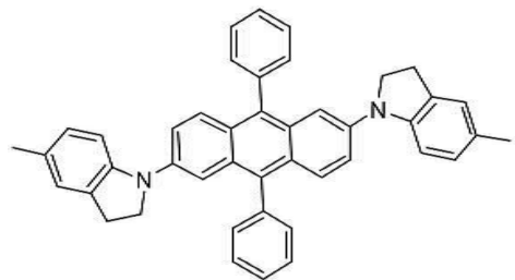
[화합물 73]
