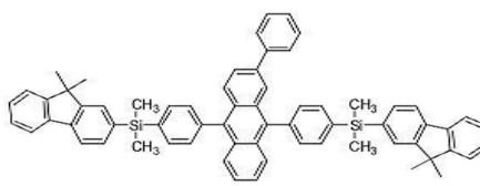
[화합물 46]
