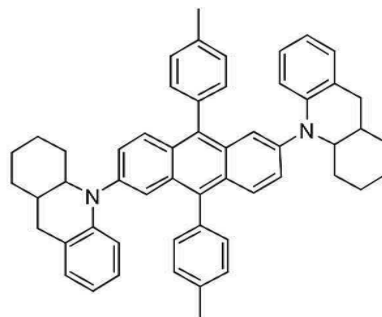
[화합물 110]
