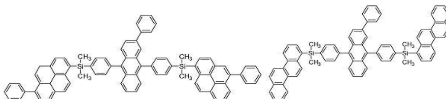
[화합물 39]
