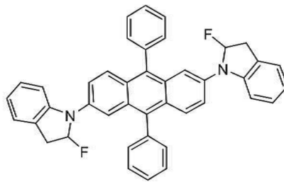
[화합물 70]
