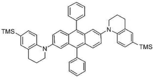
[화합물 89]
