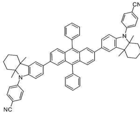
[화합물 128]
