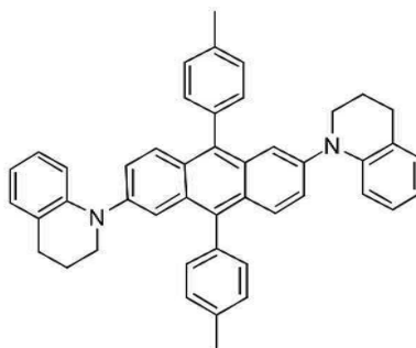
[화합물 80]
