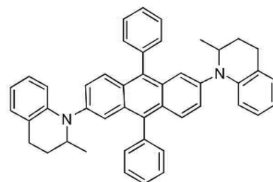
[화합물 81]
