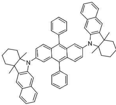
[화합물 106]
