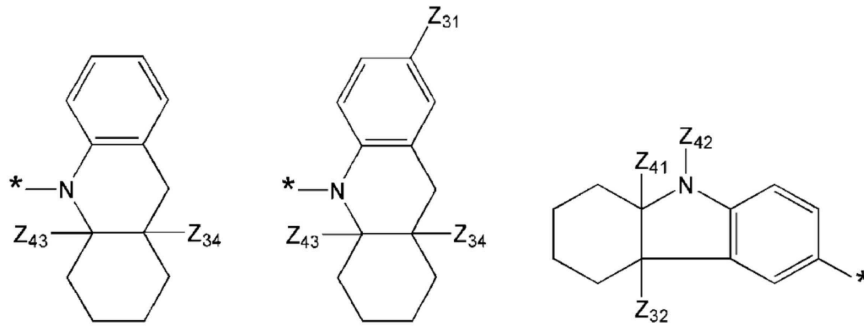
<화학식 7F(1)>
