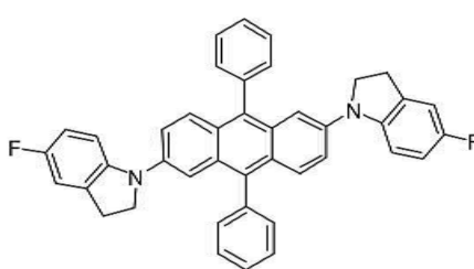
[화합물 74]
