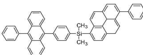
[화합물 28]
