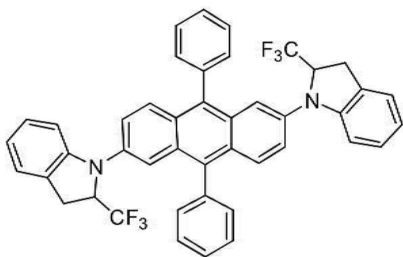
[화합물 71]
