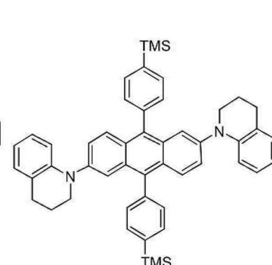
[화합물 80]
