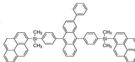
[화합물 54]
