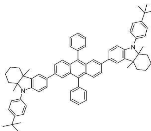
[화합물 124]
