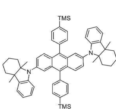
[화합물 98]
