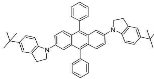
[화합물 74]
