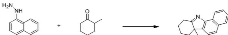
화합물 103-1
