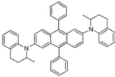
[화합물 83]
