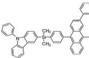
[화합물 51]
