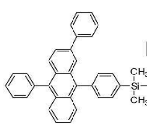
[화합물 61]
