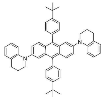
[화합물 79]
