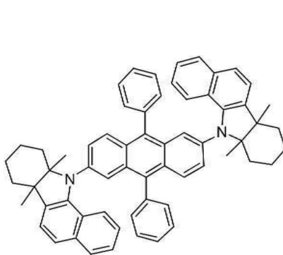
[화합물 105]
