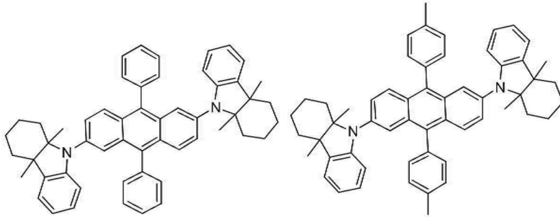
[화합물 95]
