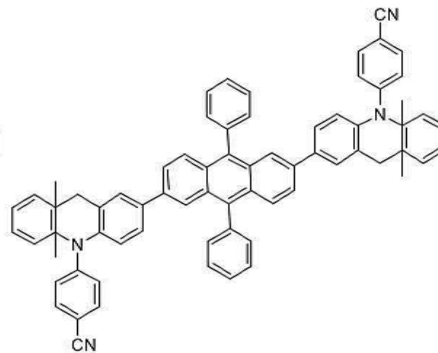
[화합물 136]
