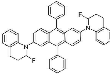
[화합물 86]
