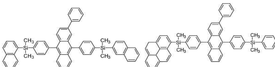
[화합물 37]
