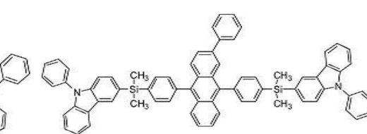
[화합물 52]
