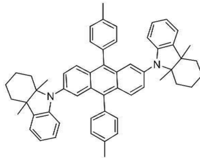
[화합물 96]
