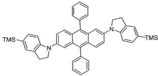
[화합물 75]
