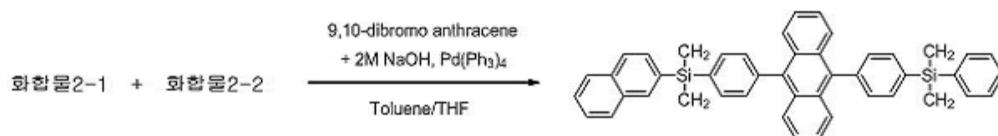
화합물 2
