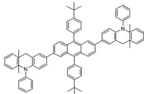
[화합물 129]
