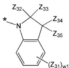
<화학식 7C>
