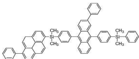
[화합물 39]
