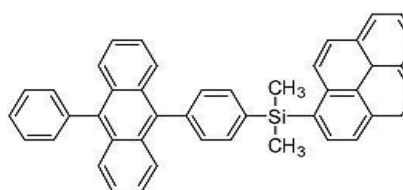
[화합물 27]
