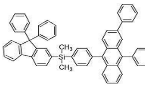
[화합물 49]
