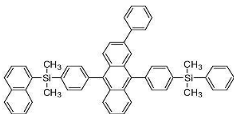
[화합물 33]
