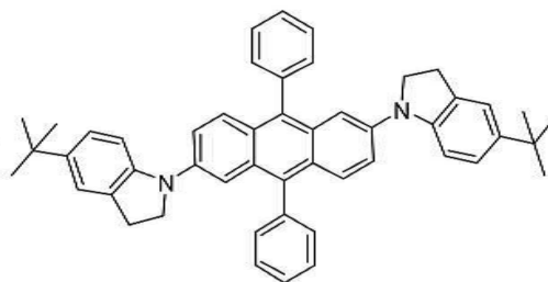
[화합물 74]
