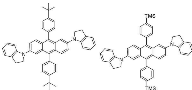
[화합물 65]
