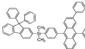
[화합물 47]
