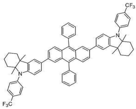
[화합물 127]
