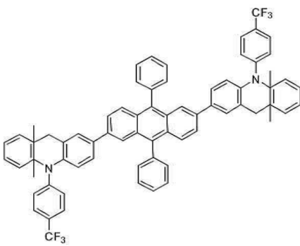
[화합물 135]
