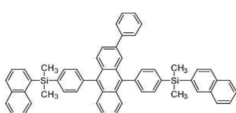
[화합물 37]
