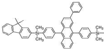
[화합물 45]
