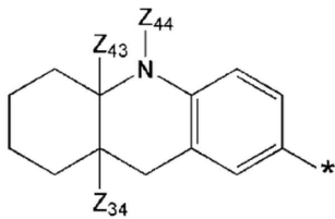
<화학식 7F(1)>
