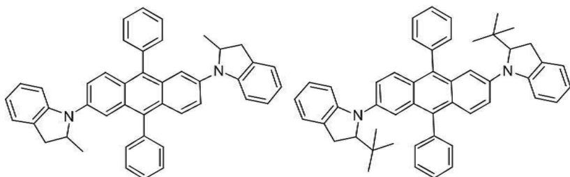
[화합물 67]
