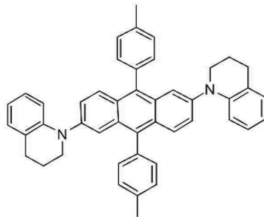
[화합물 80]
