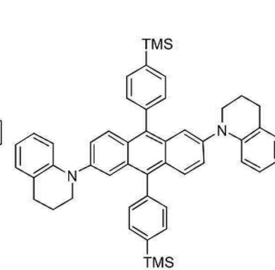
[화합물 82]
