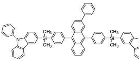
[화합물 51]
