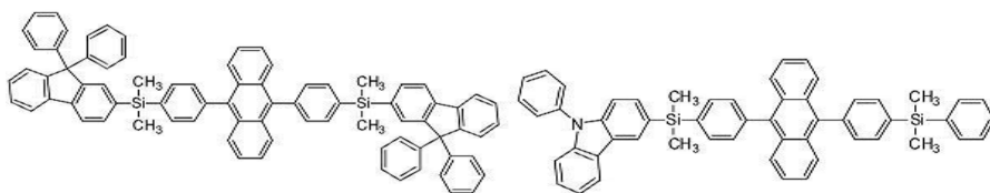
[화합물 19]
