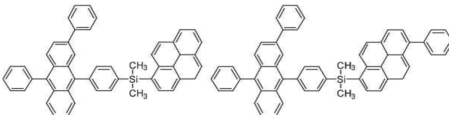
[화합물 57]
