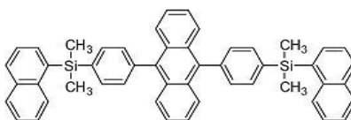
[화합물 5]
