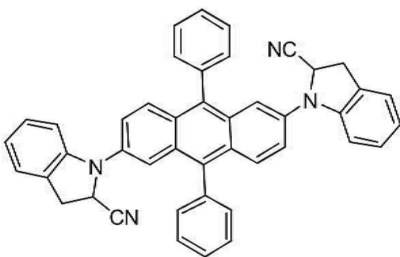
[화합물 72]
