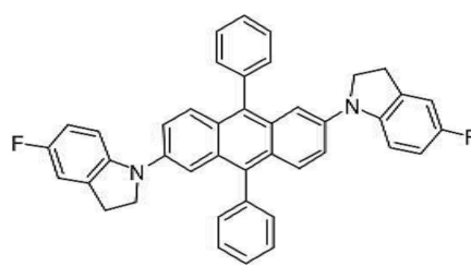
[화합물 74]
