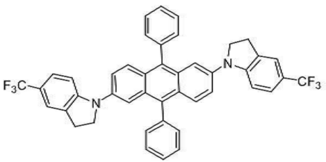
[화합물 77]
