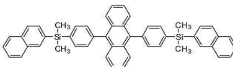
[화합물 6]
