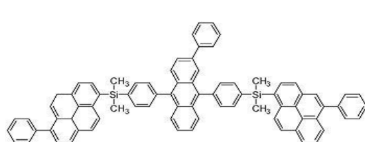
[화합물 41]
