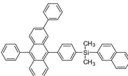
[화합물 54]
