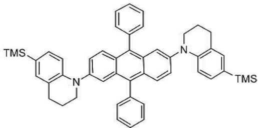
[화합물 91]
