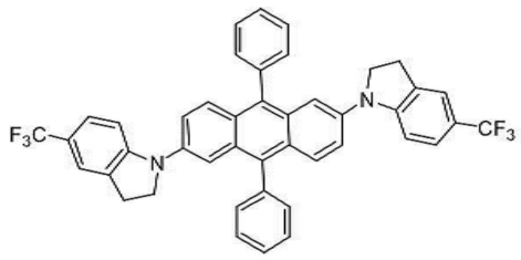
[화합물 77]
