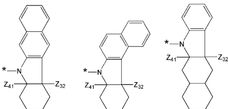
<화학식 7D(1)> <화학식 7D(2)> <화학식 7E(1)>
