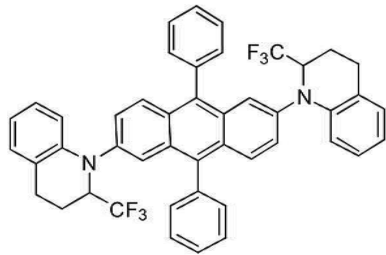
[화합물 87]
