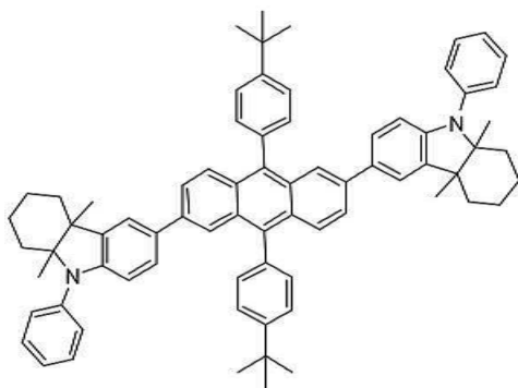
[화합물 121]
