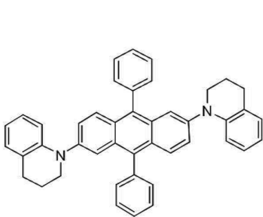
[화합물 79]
