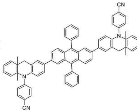
[화합물 136]
