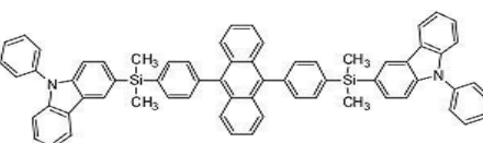
[화합물 22]
