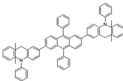
[화합물 129]
