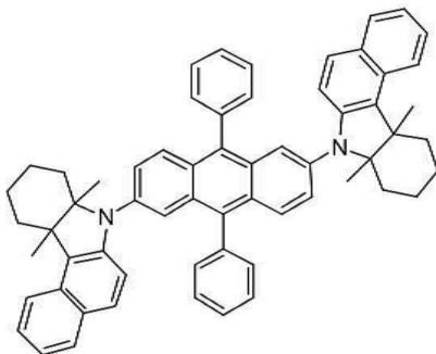
[화합물 105]
