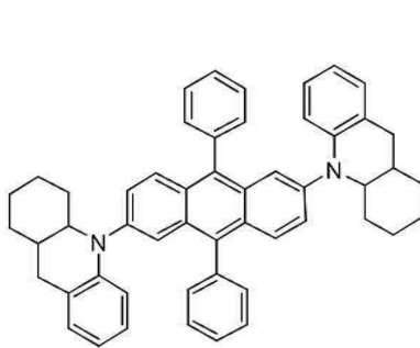
[화합물 109]
