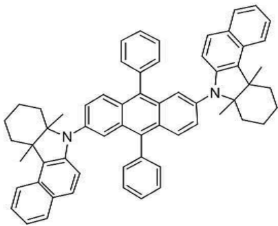
[화합물 107]
