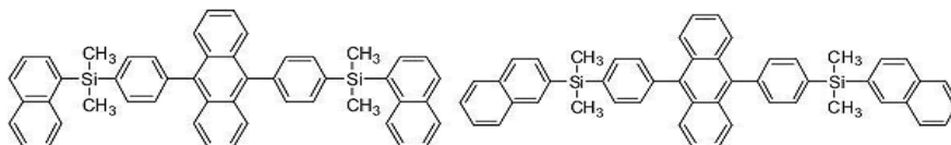
[화합물 5]
