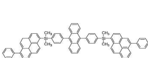
[화합물 11]
