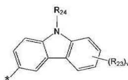
화학식 4E
