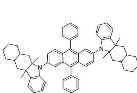
[화합물 106]
