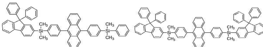
[화합물 17]
