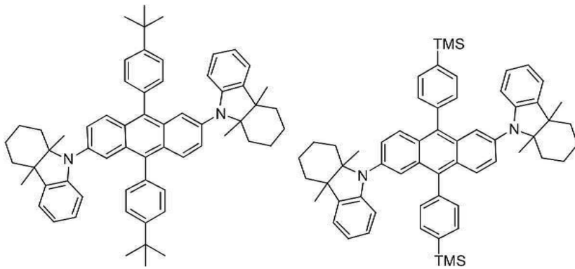
[화합물 97]
