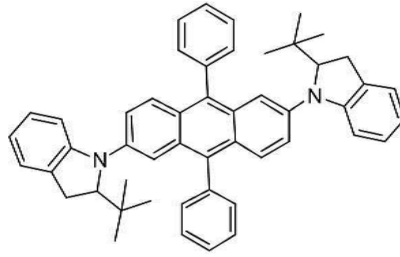
[화합물 68]
