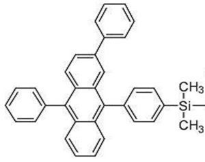
[화합물 57]
