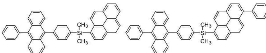
[화합물 27]
