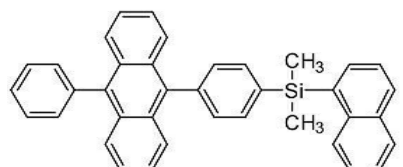
[화합물 25]
