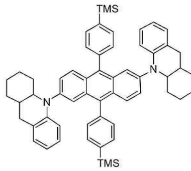
[화합물 112]
