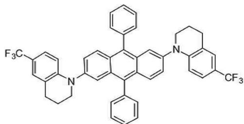
[화합물 93]
