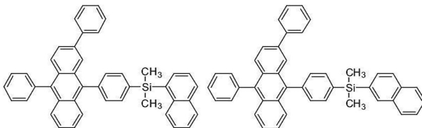
[화합물 55]
