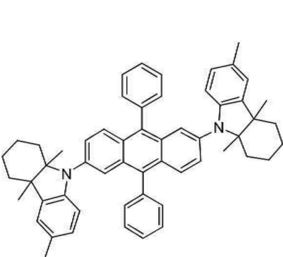
[화합물 99]
