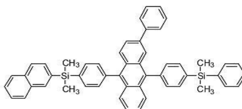
[화합물 34]
