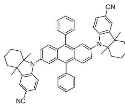
[화합물 104]
