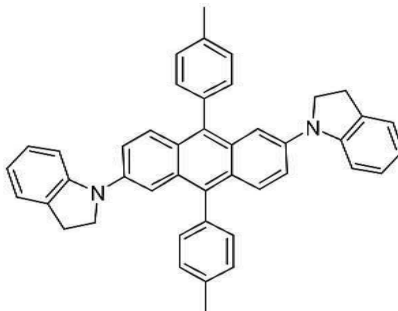
[화합물 64]
