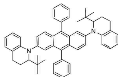
[화합물 82]
