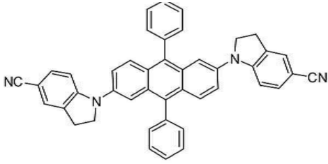
[화합물 78]
