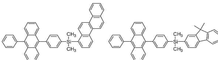
[화합물 29]
