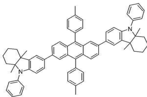
[화합물 120]
