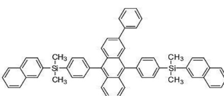
[화합물 36]
