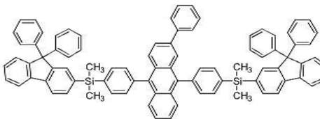
[화합물 48]
