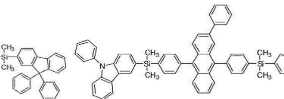
[화합물 50]
