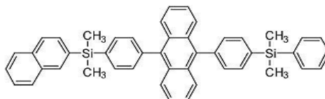
[화합물 4]
