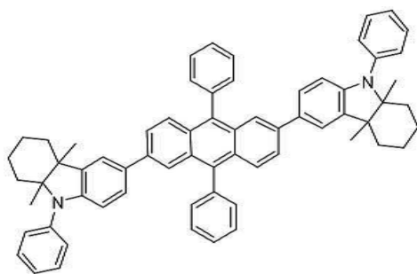
[화합물 119]
