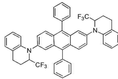
[화합물 87]
