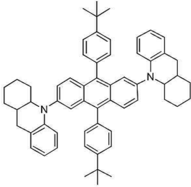
[화합물 111]
