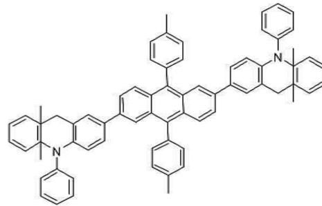
[화합물 132]
