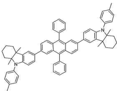
[화합물 123]
