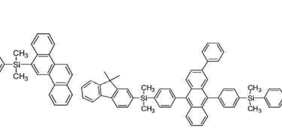
[화합물 44]
