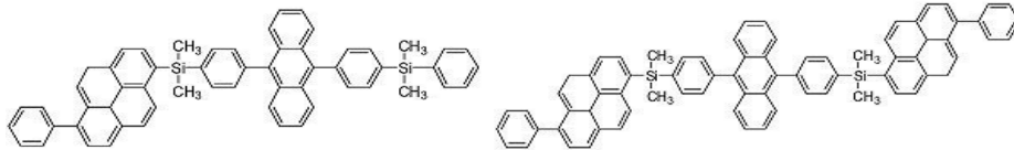
[화합물 9]
