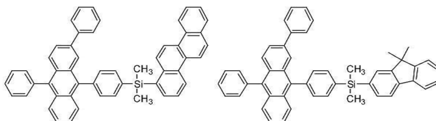
[화합물 59]
