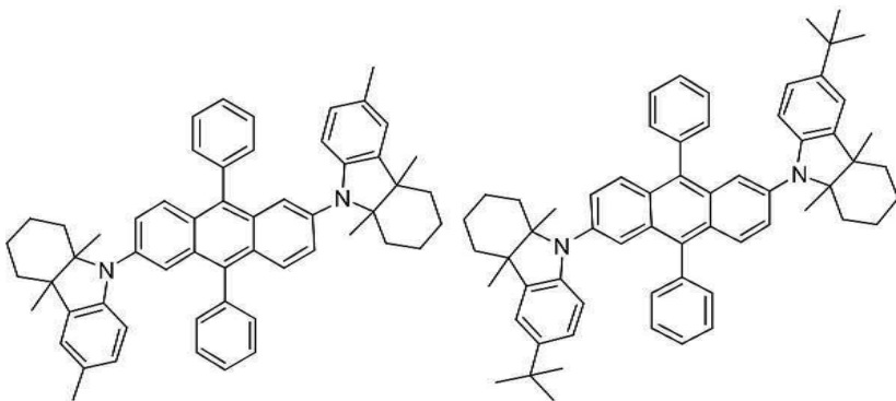
[화합물 99]
