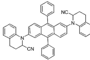
[화합물 88]
