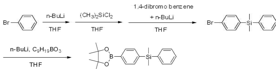
화합물 2-1
