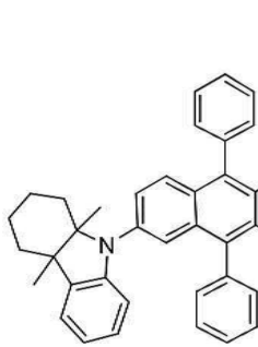
[화합물 95]
