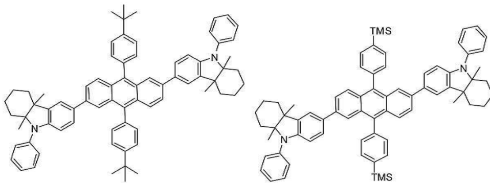
[화합물 121]
