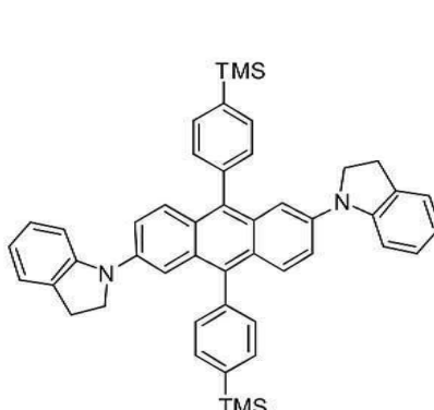
[화합물 64]
