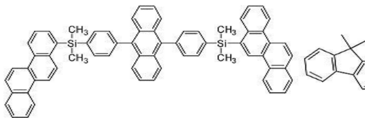
[화합물 13]
