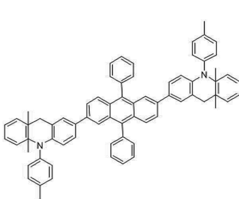
[화합물 131]
