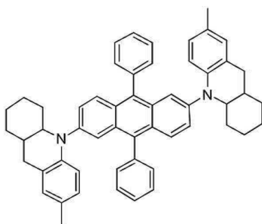
[화합물 113]
