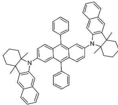
[화합물 106]
