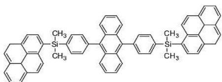
[화합물 23]
