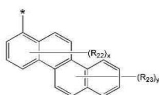
화학식 4I
