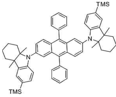
[화합물 101]
