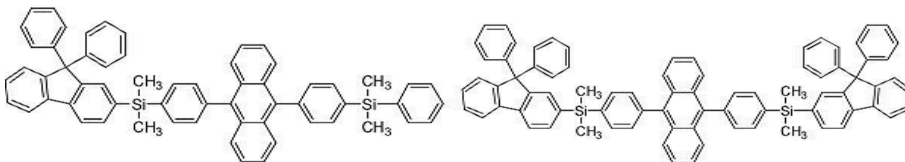
[화합물 17]
