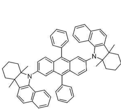
[화합물 105]
