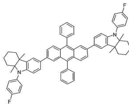
[화합물 124]
