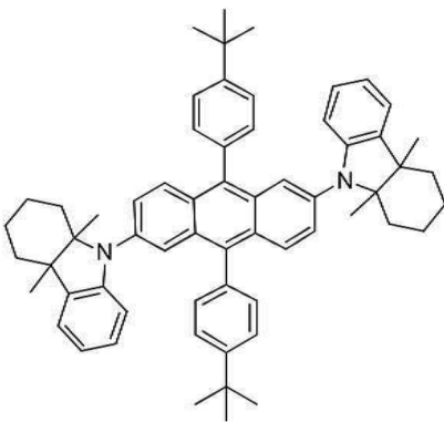
[화합물 97]
