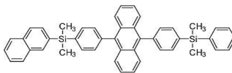
[화합물 4]
