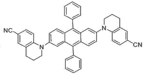
[화합물 94]
