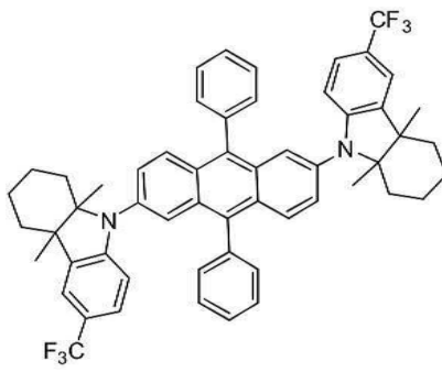
[화합물 103]
