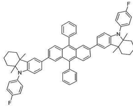
[화합물 126]
