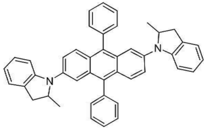
[화합물 67]
