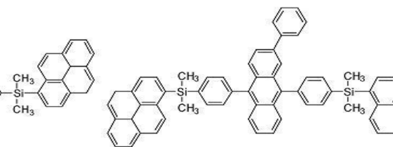
[화합물 54]
