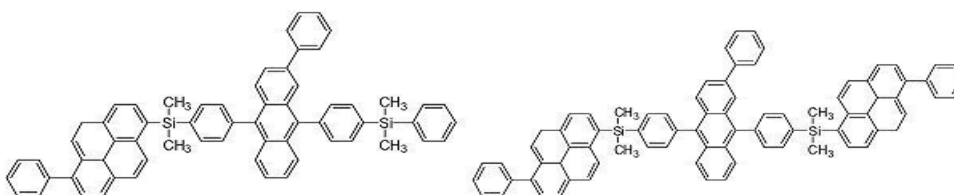
[화합물 39]
