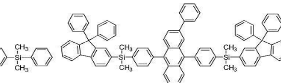
[화합물 48]
