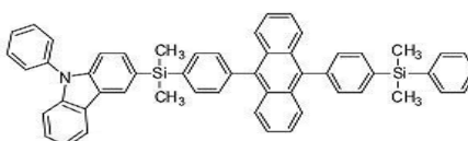
[화합물 20]
