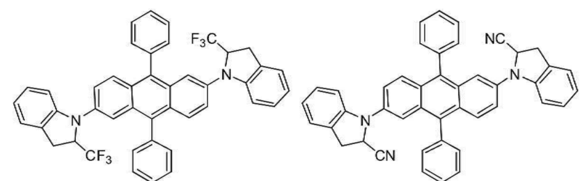
[화합물 69]
