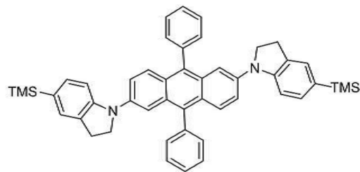
[화합물 73]
