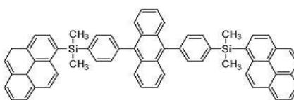
[화합물 24]
