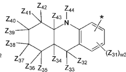
<화학식 7F>
