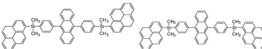
[화합물 23]
