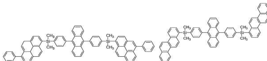
[화합물 11]
