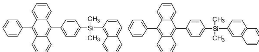
[화합물 25]
