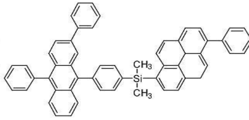
[화합물 58]
