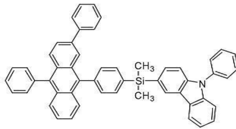
[화합물 60]
