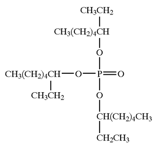
Solvent CS-3
