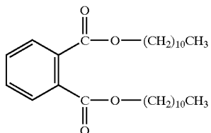
Solvent CS-2
