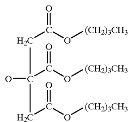
Solvent CS-1
