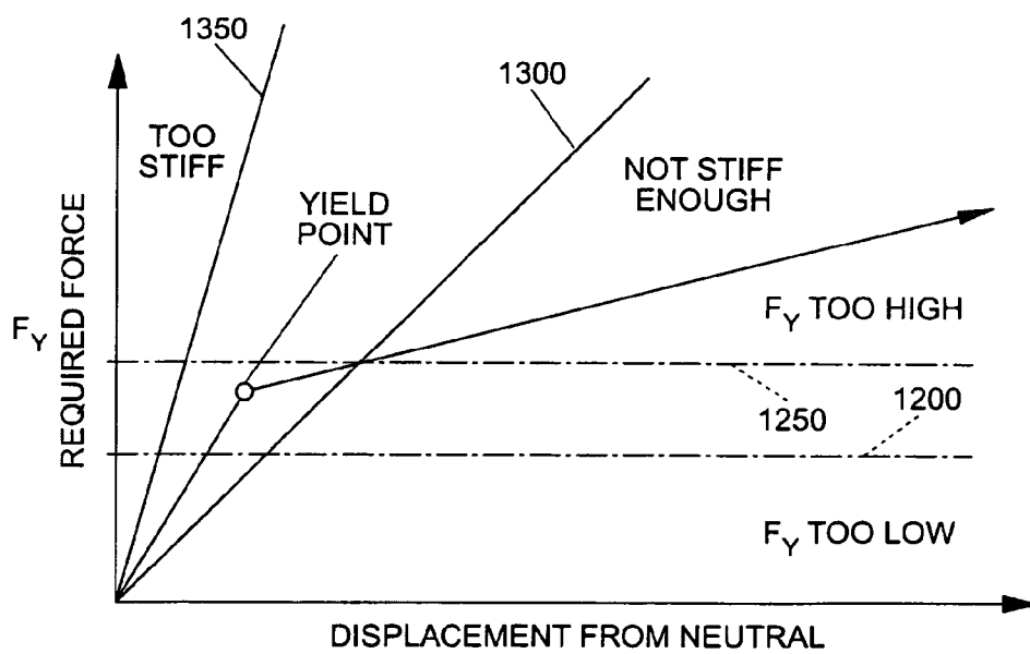
FIG. 23
