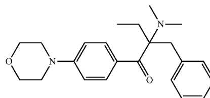
Irgacure 369 (BASF)
