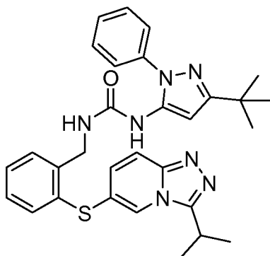
Y1W 1-(3-tert-butyl-1-phenyl-1H-pyrazol-5-yl)-3-(2-([3-(1-methylethyl)[1,2,4]triazolo[4,3-a]pyridine-6-yl]sulfanyl)benzyl)urea
