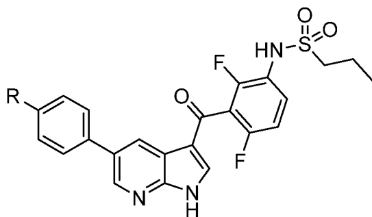
PLX4032
