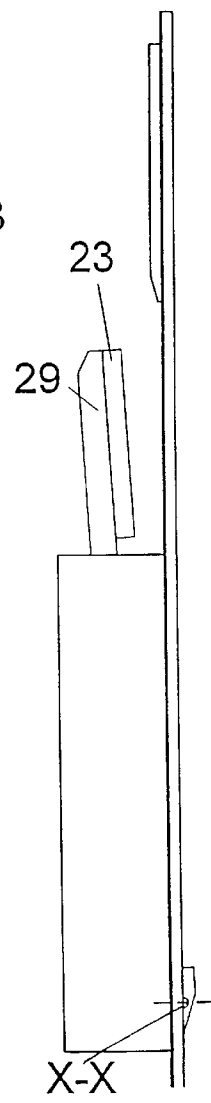
Fig. 6
