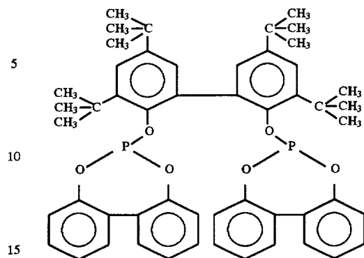
Ligand D
