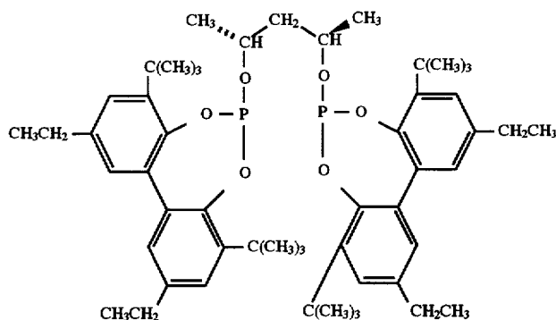
Ligand L
