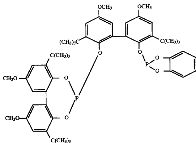
Ligand O
