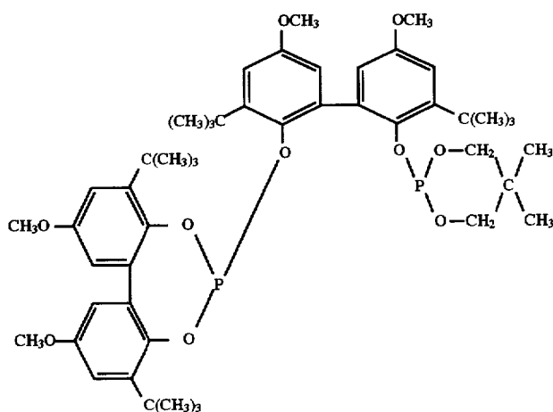
Ligand P
