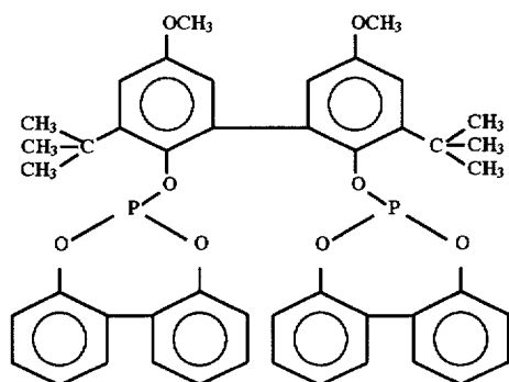
Ligand D
