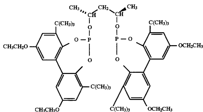
Ligand K
