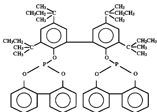
Ligand E
