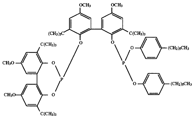
Ligand Q
