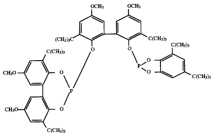
Ligand N
