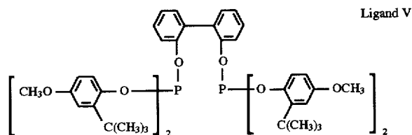
Ligand V
