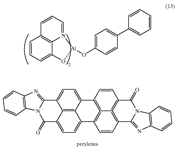
Alq3
