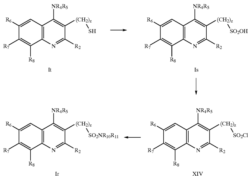
SCHEME VI
