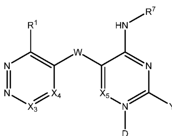
Formula 1i.
