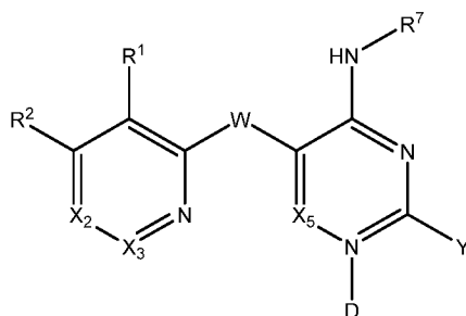
Formula 1e.
