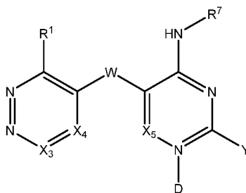
Formula 1i.
