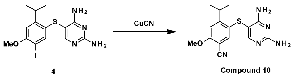
Scheme N:
