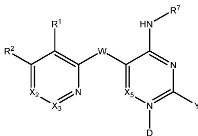
Formula 1e.
