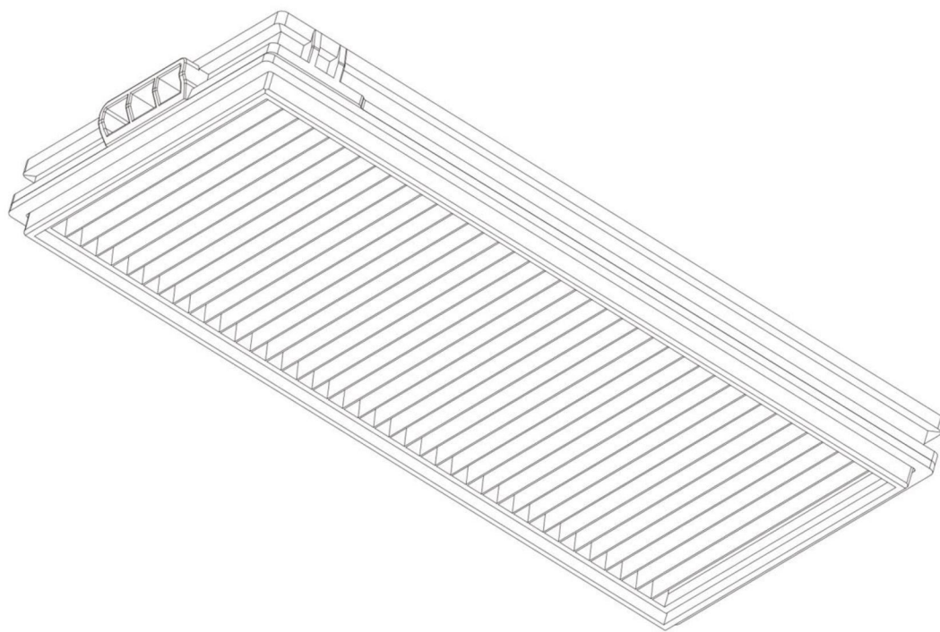
立體圖 2
