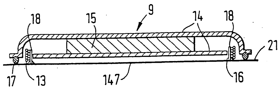
Fig. 11c
