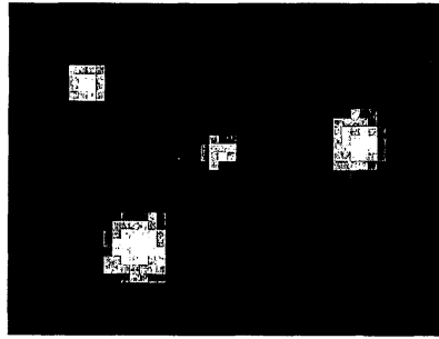
필터링된 데이터
