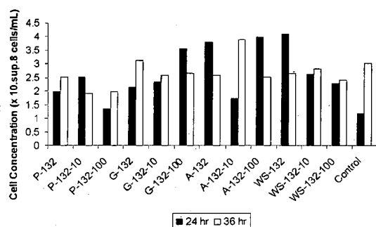
Chart 3A. Cell Concentrations for S. cerevisiae
