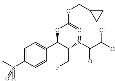
Cyclopropylmethyl(1R,2S)-2-(2,2-dichloroacetamido)-3-fluoro-1-(4-(methylsulfonyl)phenyl)propyl carbonate
