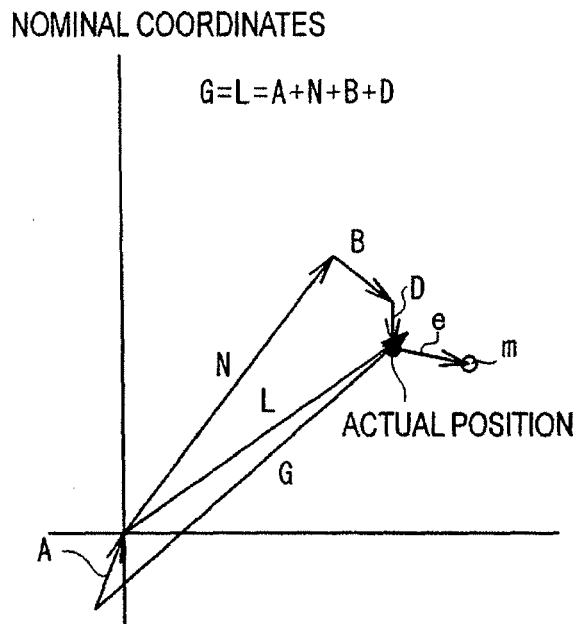
FIG. 17A
