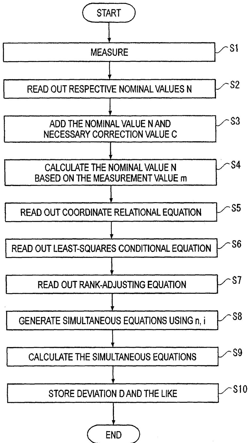
FIG. 21
