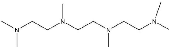
1,1,4,7,10,10六甲基三乙四胺
