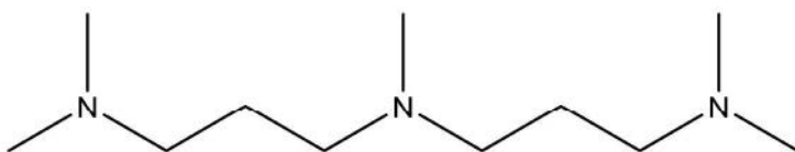
2,6,10,三甲基2,6,10三氮杂十一烷
