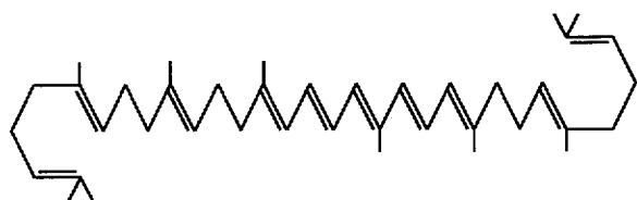
PHYTOFLUENE
