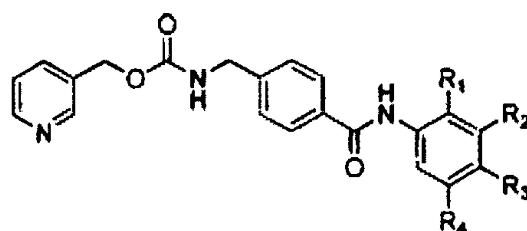
MS-275
