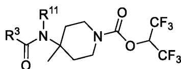
Formula (IIa);
